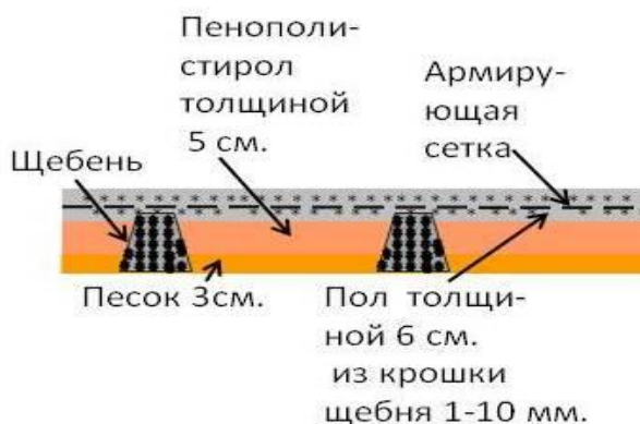
Рис. 4 Полы в доме
