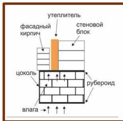
Рис. 8 Стена дома с цоколем.
