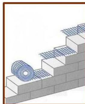
Рис. 15 Армирование рядов блока
