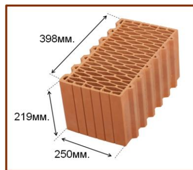
Рис. 19 Керамический блок 398х250х219
