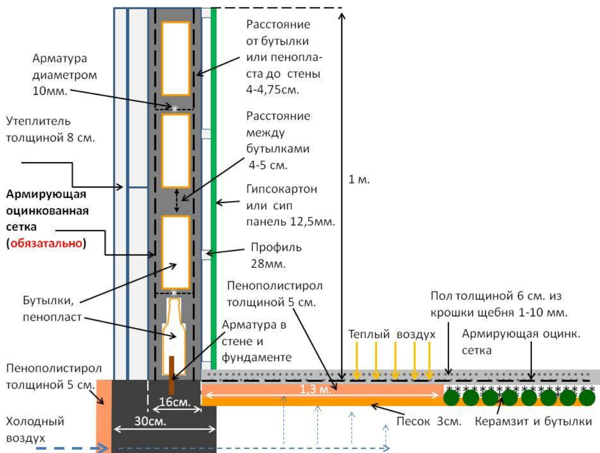
Рис. 10 Пол и стена «КоПалыч» в разрезе вид с боку
