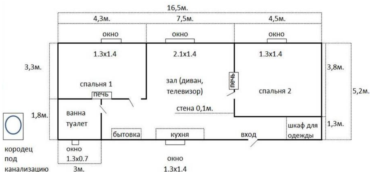
Рис. 2 Длинна стен дома считается с учётом ширины внутренних стенок в 10см.
