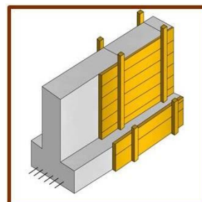
Рис. 9 Щитовая опалубка Опалубку для стен делайте с геометрической точностью. Тогда облицовка стен не займет много времени.
