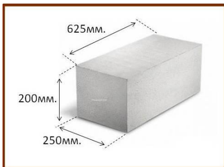
Рис. 16 Газосиликат
