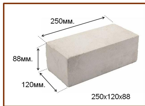
Рис. 22 Силикатный кирпич
